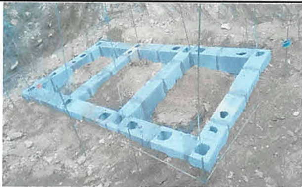
FOTO 1: LOS SANITARIOS ANTERIORES NO CONTABAN CON BASE SOLIDA, AHORA TIENE ZAJENO PROFUNDO DE DONDE VIENE EL CIMIENTO CORRIDO FUNDIDO DE CONCRETO Y ARMADO CON HIERRO DE
