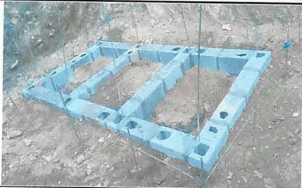
FOTO 1: LOS SANITARIOS ANTERIORES NO CONTABAN CON BASE SOLIDA, AHORA TIENE ZAJENO PROFUNDO DE DONDE VIENE EL CIMENTO CORRIDO FUNDIDO DE CONCRETO Y ARMADO CON HIERRO DE
